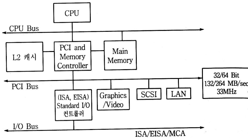
[그림 19-5] PCI 버스 구조
