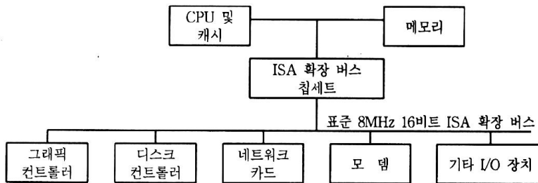
[그림 19-2] ISA 버스의 블록도
